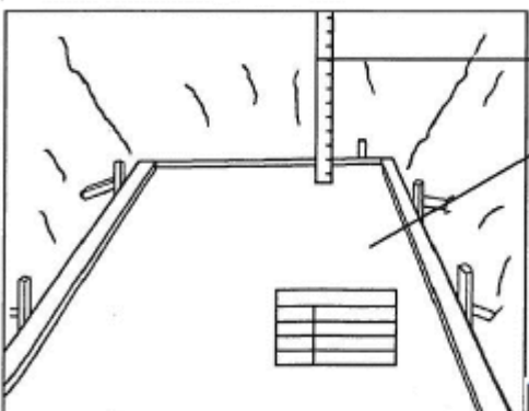
【写真4】 栗石地業後の基礎底板コンクリートを打った写真
