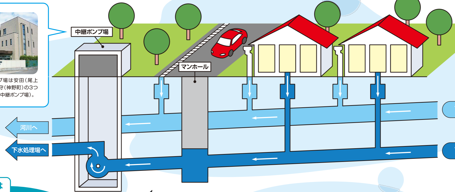
雨水が流れる「 雨水ます 」も。こちらは四角形のものもあります 汚水ますのふたの素材は塩ビや鋳物、コンクリートなどさまざまです
