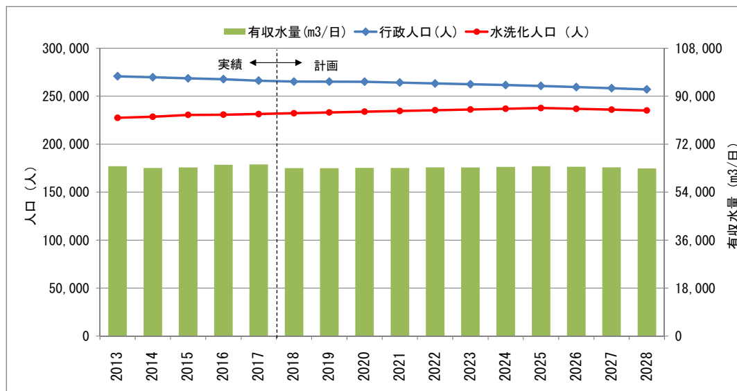
図 4.1 水洗化人口・有収水量の将来見通し
