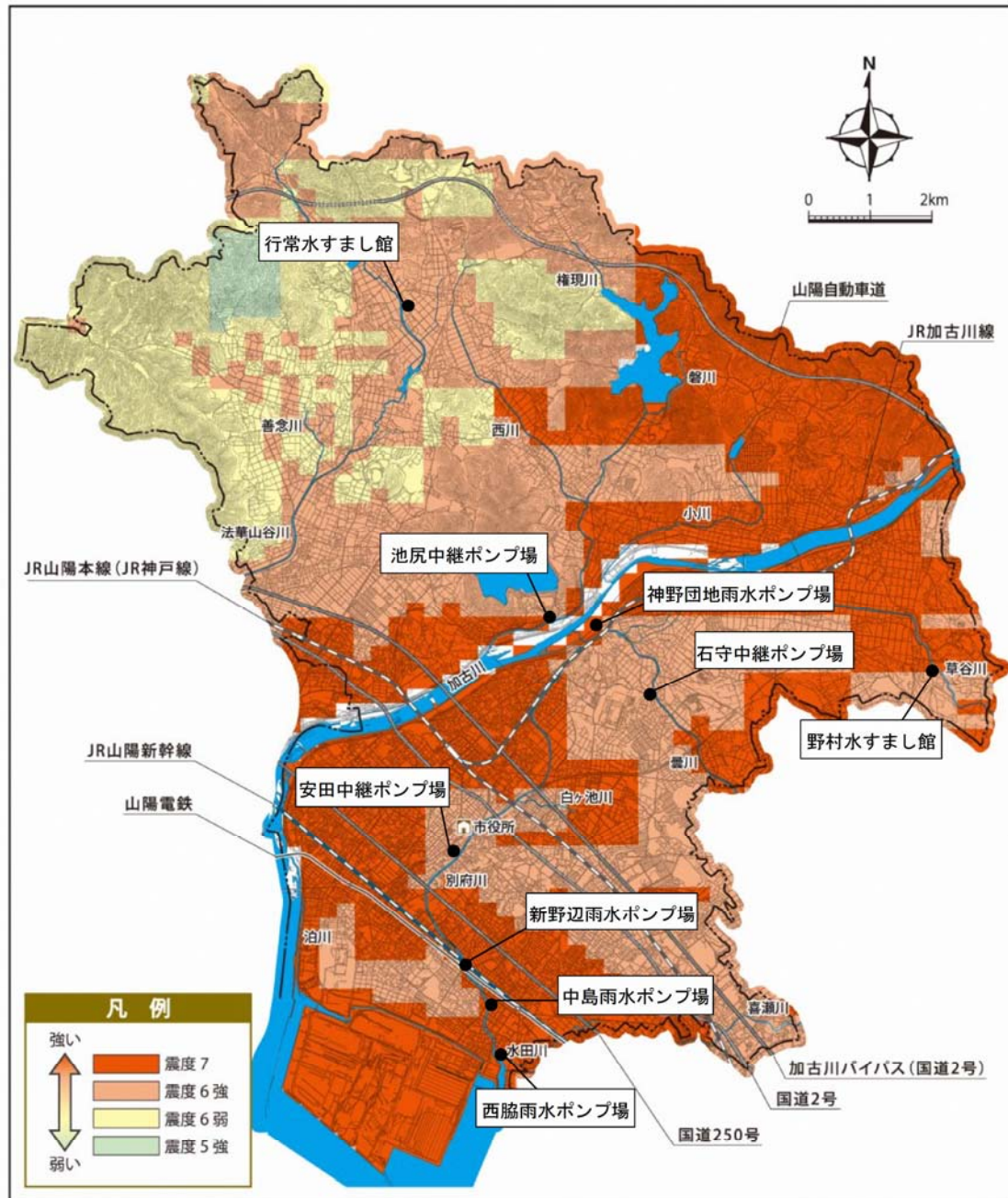
図 3.5 山崎断層帯（主部南東部・草谷断層）地震の震度分布図 出典）加古川市総合防災マップ
