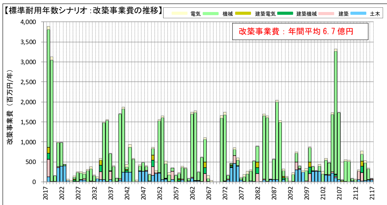
図 3.11 標準耐用年数で改築した場合のポンプ場施設の健全率と改築事業費との推移
