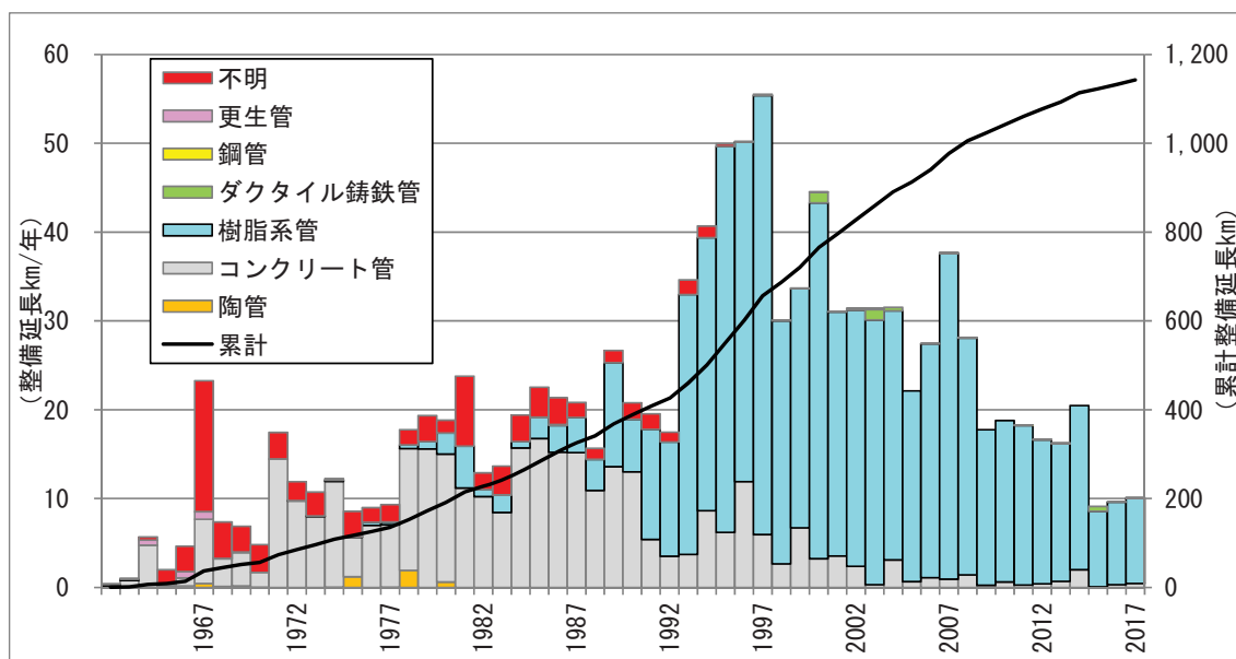
図 3.8 年度別管渠延長の推移（管種別）
