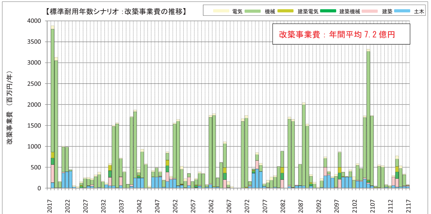
図 3.11 標準耐用年数で改築した場合のポンプ場施設の健全率と改築事業費との推移 注)改築事業費は今後 50 年間の平均値を示す。
